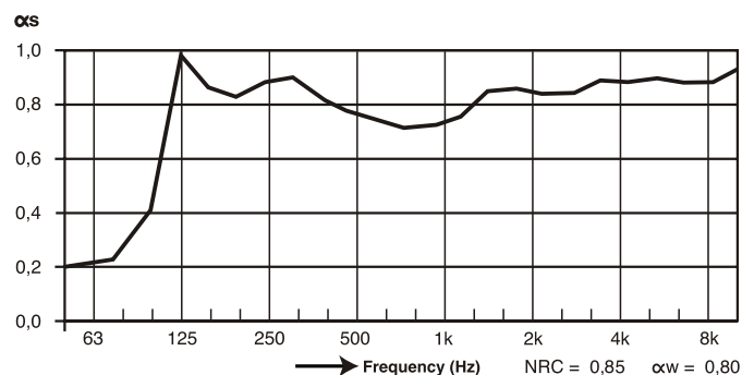
Sonacoustic® 25mm com cavidade de 125mm (TNO)
