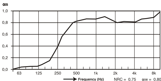
Sonacoustic® 25mm sobre base sólida (TNO)
